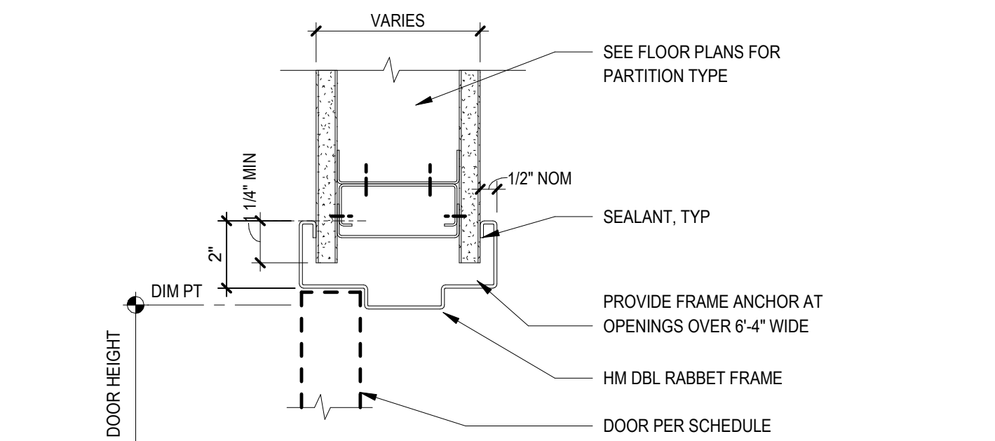
E1 FRAME TYPE: S - HM DOOR HEAD 3" = 1'-0"
