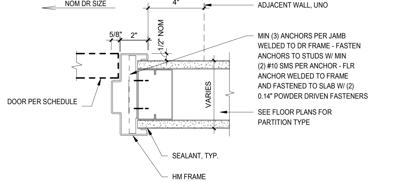
E2 FRAME TYPE: S - HM DOOR JAMB 3" = 1'-0"
